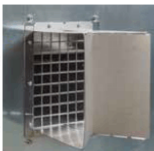
воздухораспределительная камера с двумя выходами (левый и правый)
